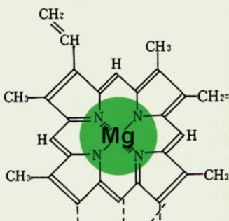
叶绿素分子结构
