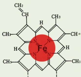
人体血液分子结构
